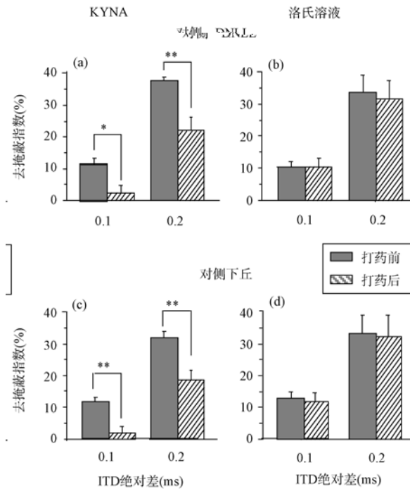
图 7 实验 3.2 中, 阻断对侧 DNLL 或对侧下丘对下丘 FFRs 双耳/空间去掩蔽的影响, * p < 0.05 , ** p < 0.01 , 配对 t 检验
